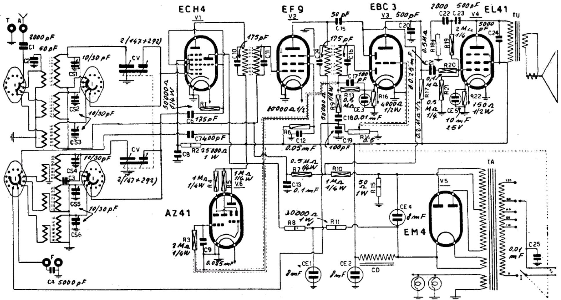
INCAR - Modd. LV 57 ed LV 501 - Gamma onde medie e due gamme onde corte. Campo dinamico di 1200 ohm. Potenza d'uscita 4 watt.
